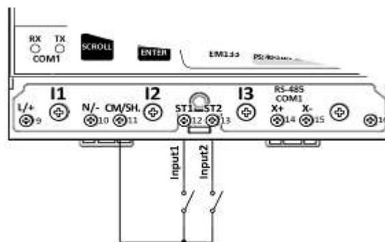
Рисунок 2-21 Подключения дискретных входов EM133
