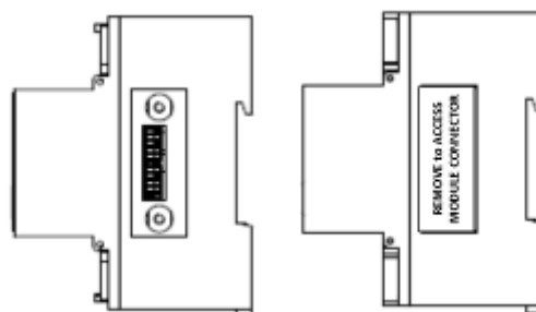
Рисунок 2-4 Расположение разъема дополнительного модуля EM133
