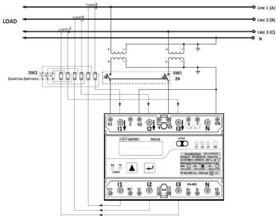
Рисунок 2-14 3-проводное соединение в разомкнутый треугольник, 2 элемента, 2 ТН, 2 ТТ (режим подключения = 3P2)
