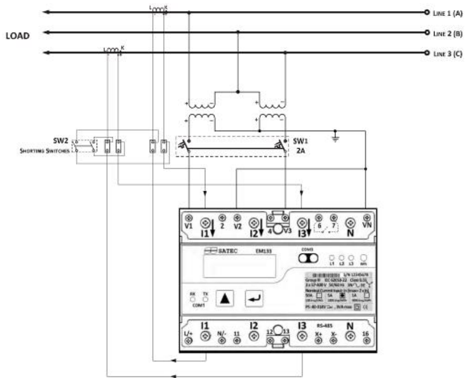
Рисунок 2-14 3-проводное соединение в разомкнутый треугольник, 2 элемента, 2 ТН, 2 ТТ (режим подключения = 3P2)
