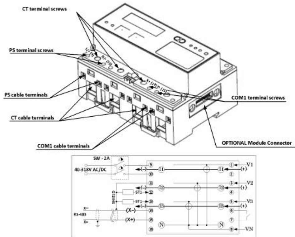
Рисунок 2-7 Схема подключения зажимов
