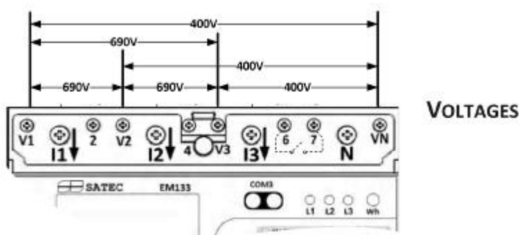
Рисунок 2-9 Подключение измеряемого напряжения к EM133
