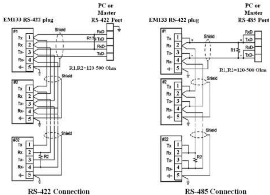
Рисунок 2-31 Подключение COM2 RS-422/485
