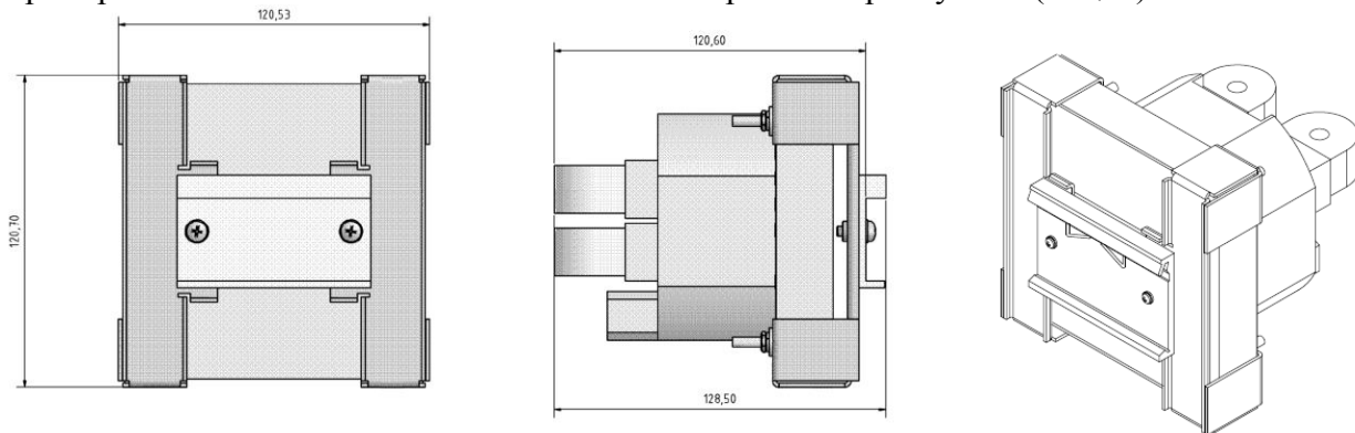
Рисунок 2-3а Монтаж PM130 PLUS на DIN-рейку
