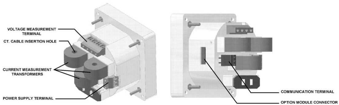
Рисунок 2-3 Монтаж PM130 PLUS
