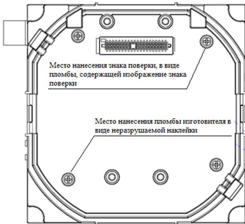
Рисунок 5-1 – Схема пломбирования счетчиков модификаций PRO PM035 и
