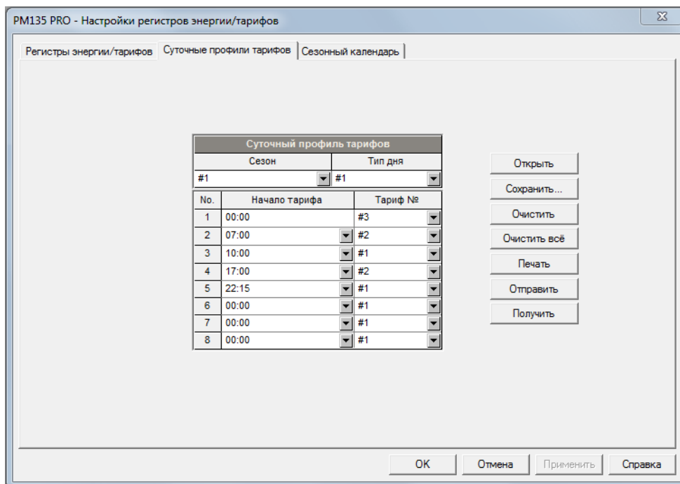
Рисунок 110 – Настройка суточных профилей тарифов
