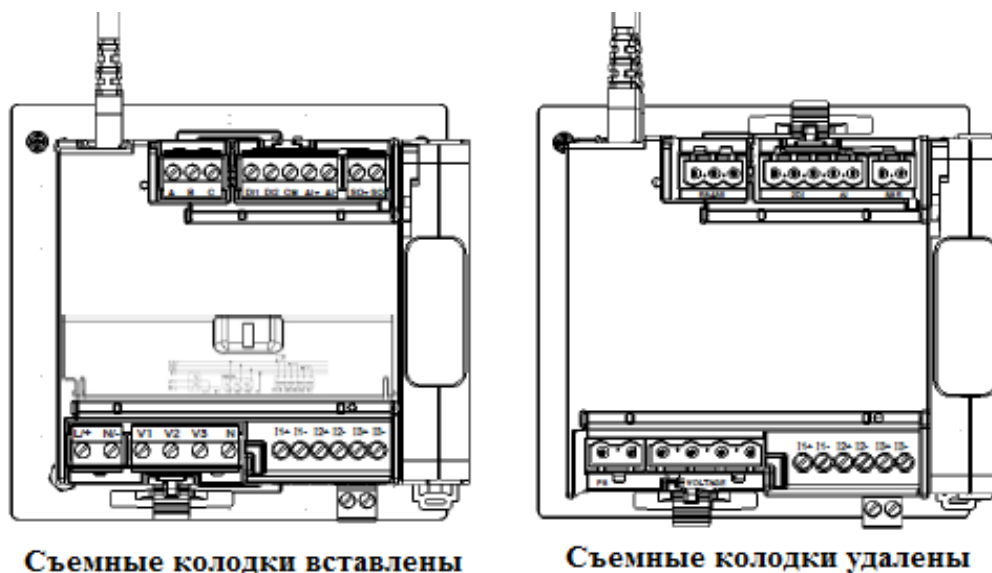
Счетчики модификаций PRO PM035, PRO PM335
