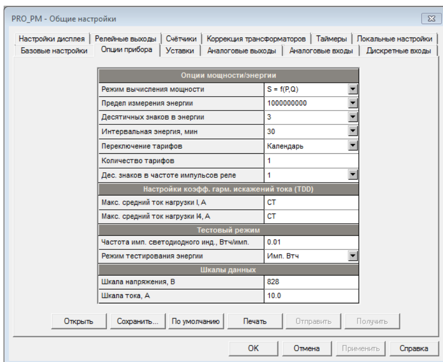
Рисунок 80 –Настройки опций счетчика
