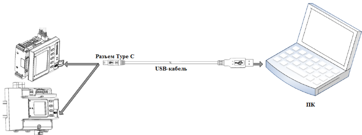
Рисунок 36 – Схема подключения USB-порта
