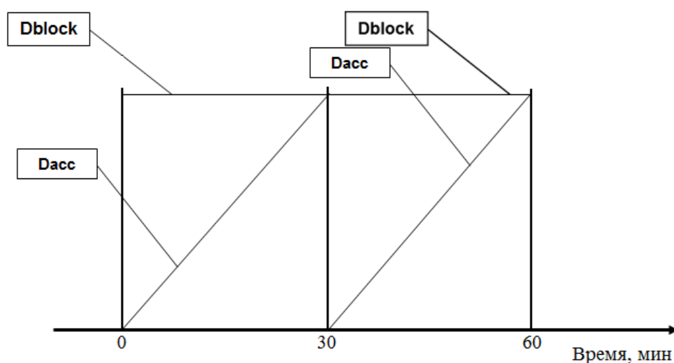
Рисунок 3 – Иллюстрация аккумулярованного профиля мощности
