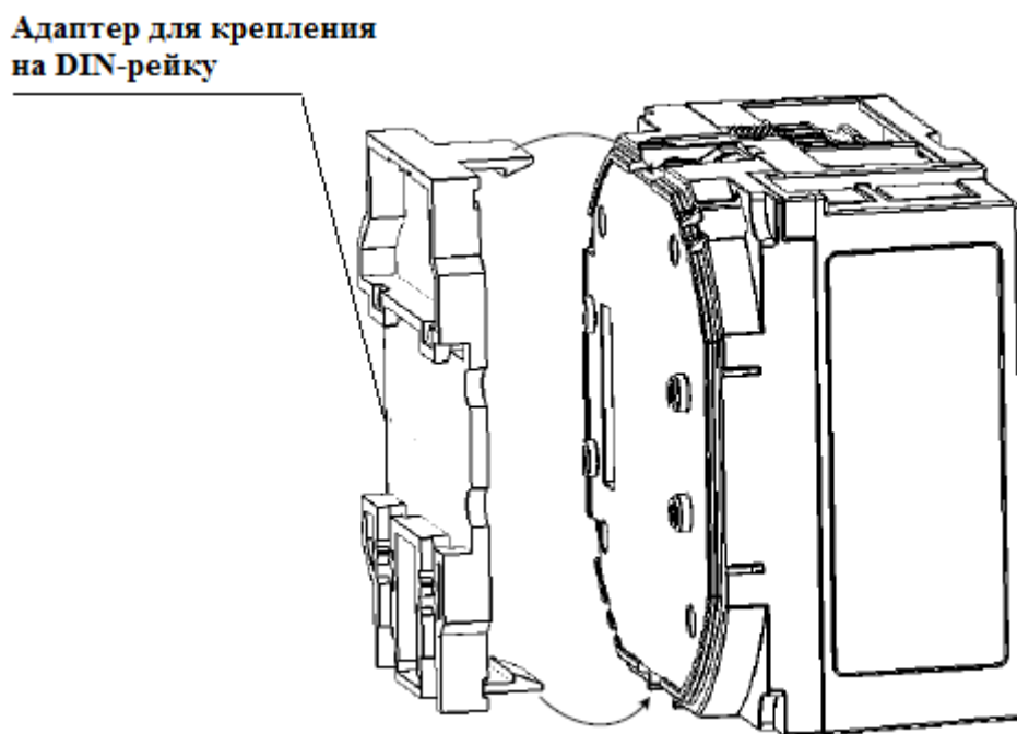
Рисунок 13 – Схема крепления адаптера для DIN-рейки
