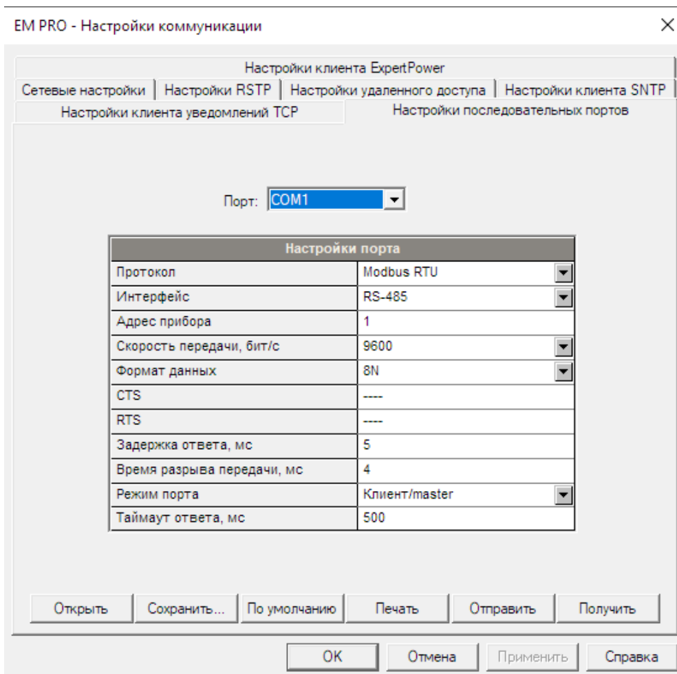
Рисунок 70 – Окно настроек параметров последовательных портов
