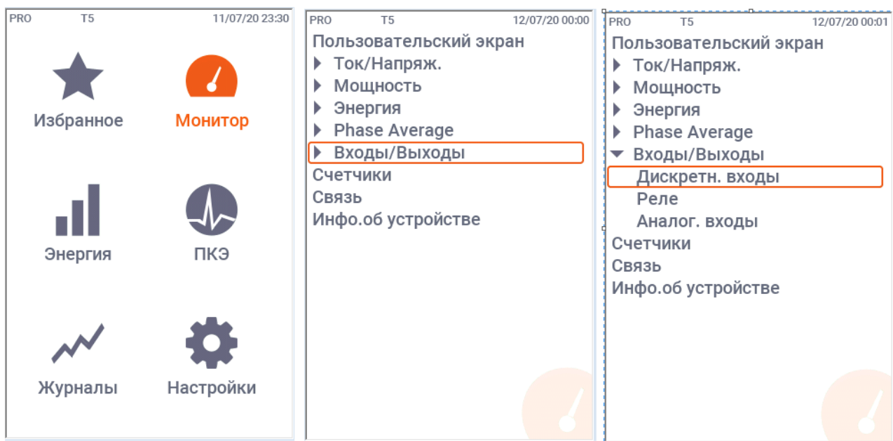
Рисунок 50 – Схема перехода к пунктам меню «Входы/Выходы»
