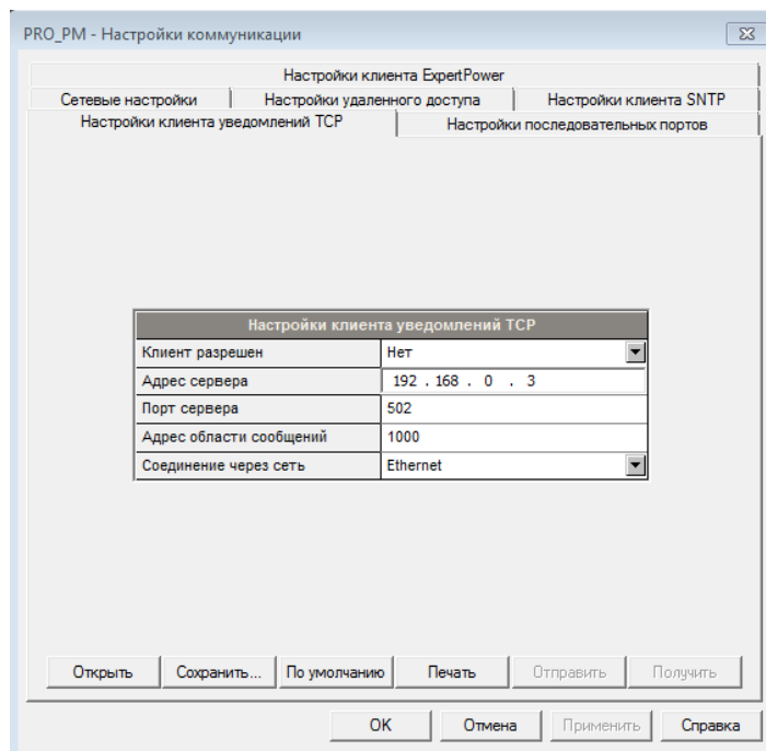
Рисунок 76 – Настройки TSP-клиента уведомлений
