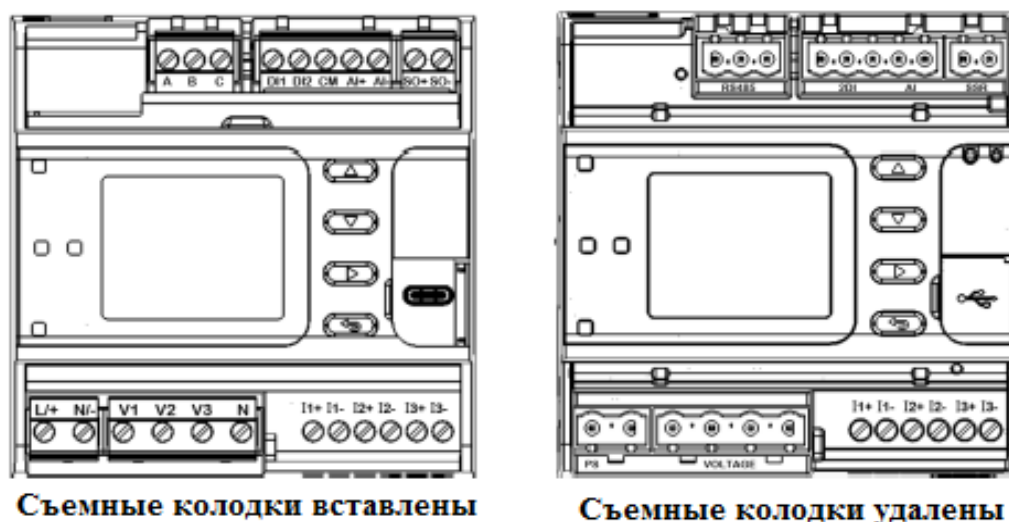
Счетчик модификации PRO EM235
