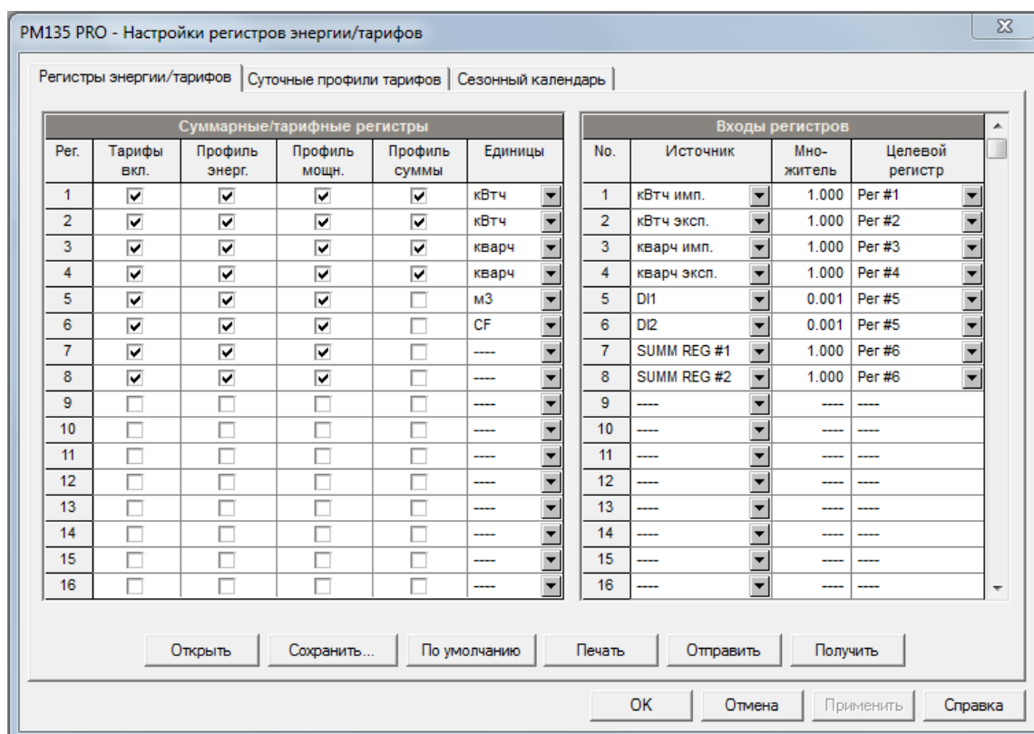
Рисунок 109 – Настройка регистров учета
