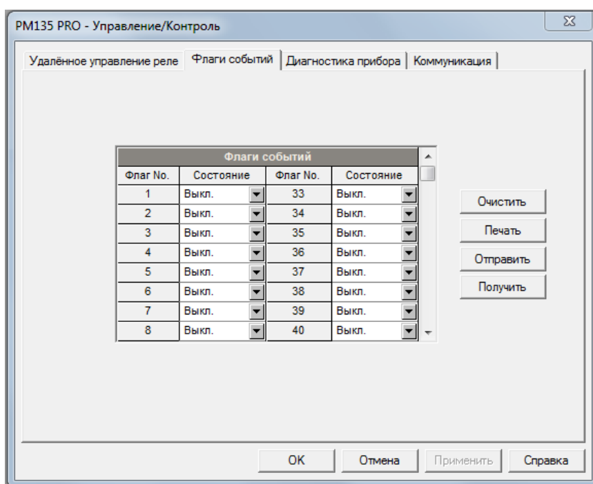
Рисунок 127 – Флаги событий
