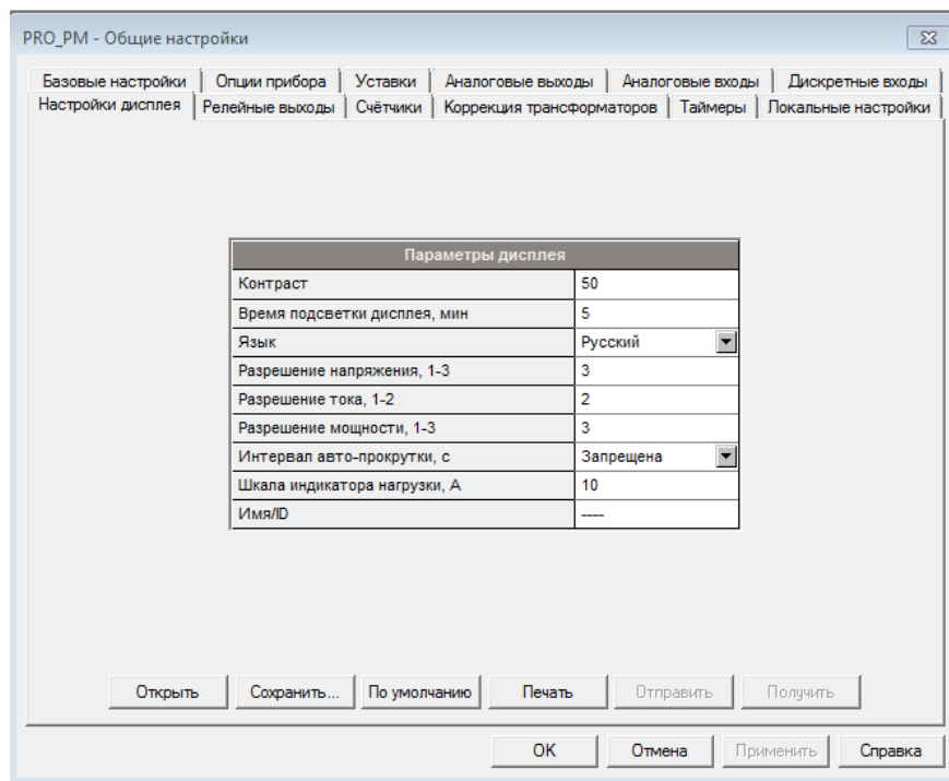
Рисунок 97 – Настройки дисплея
