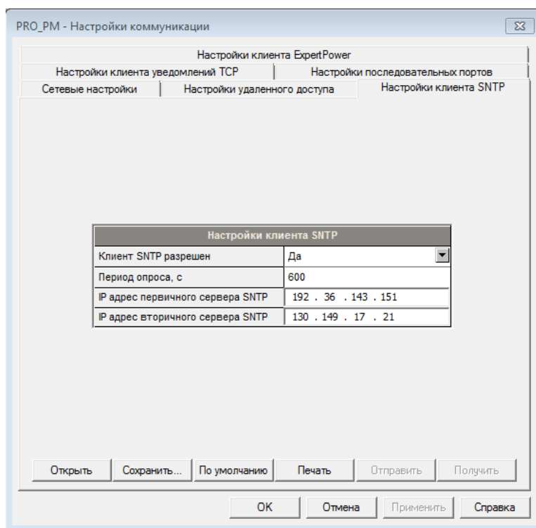
Рисунок 75 – Настройка SNTP-клиента
