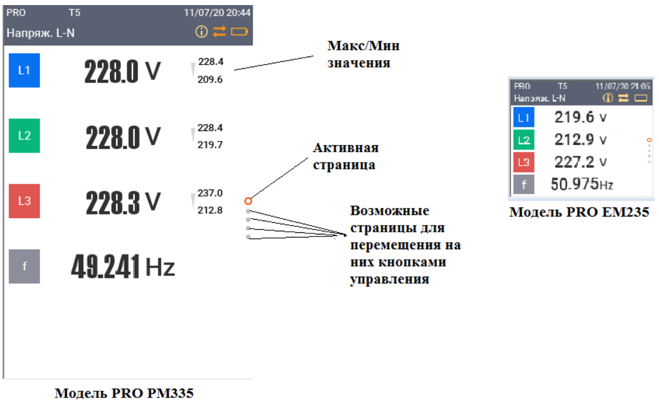
Рисунок 41 – Экран отображения данных
