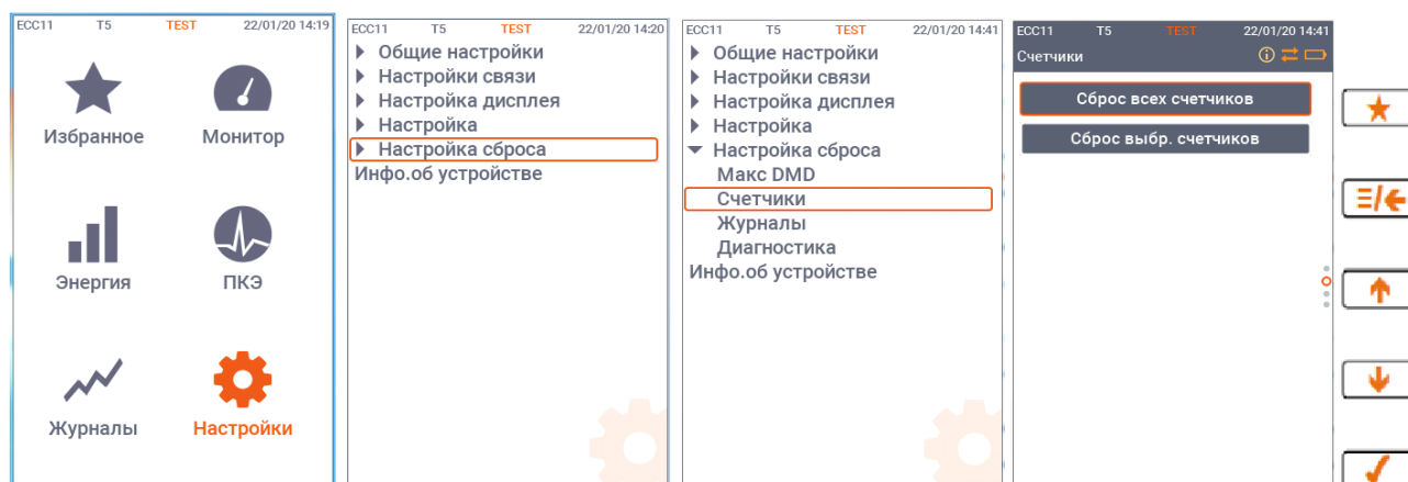
Рисунок 131 – Схема перехода к экранной форме сброса значений счетчиков импульсов (событий)
