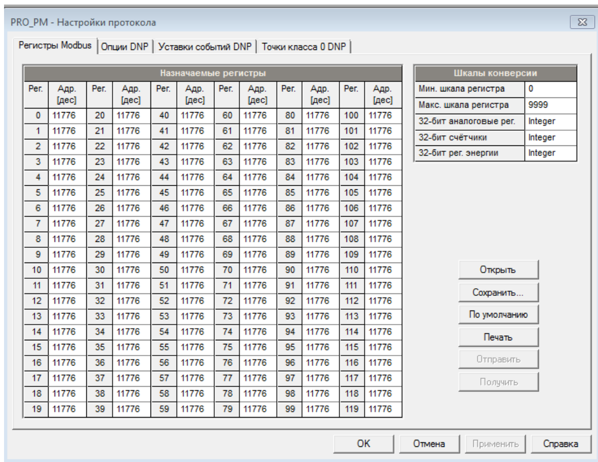
Рисунок 112 – Построение карты регистров Modbus
