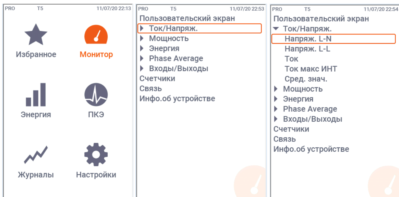
Рисунок 44 – Схема перехода к пунктам меню «Ток/Напряж»
