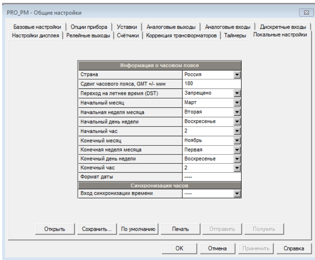
Рисунок 99 – Настройки локализации
