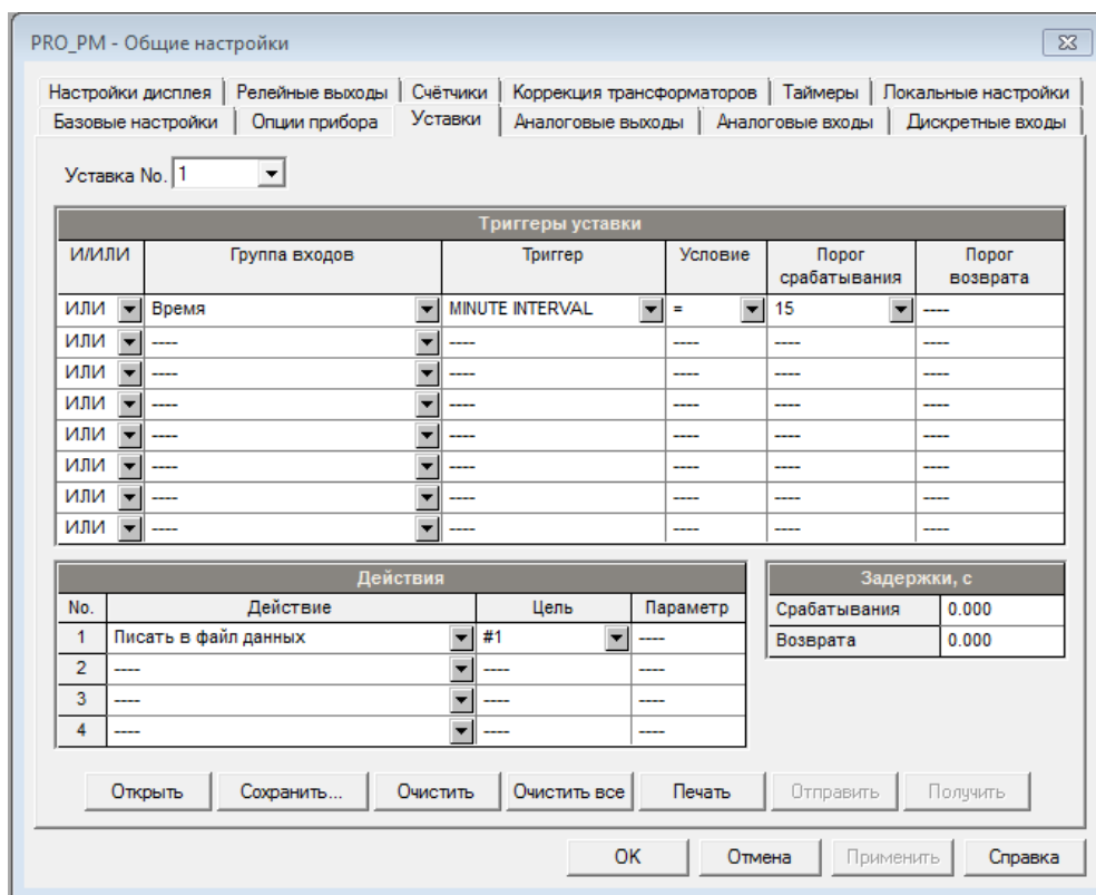
Рисунок 90 – Настройки уставок
