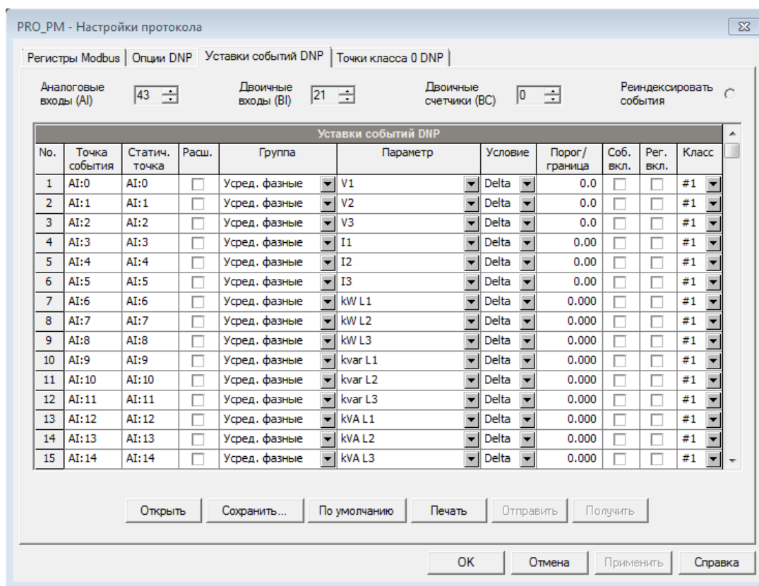
Рисунок 115 – Уставки событий DNP
