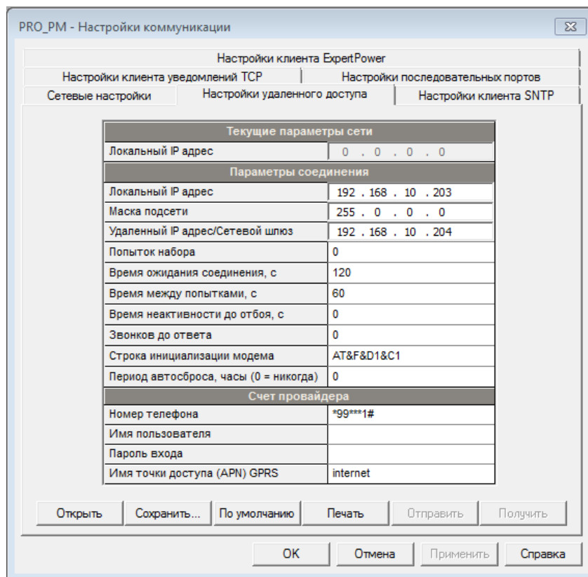
Рисунок 74 – Настройки связи по сотовой сети
